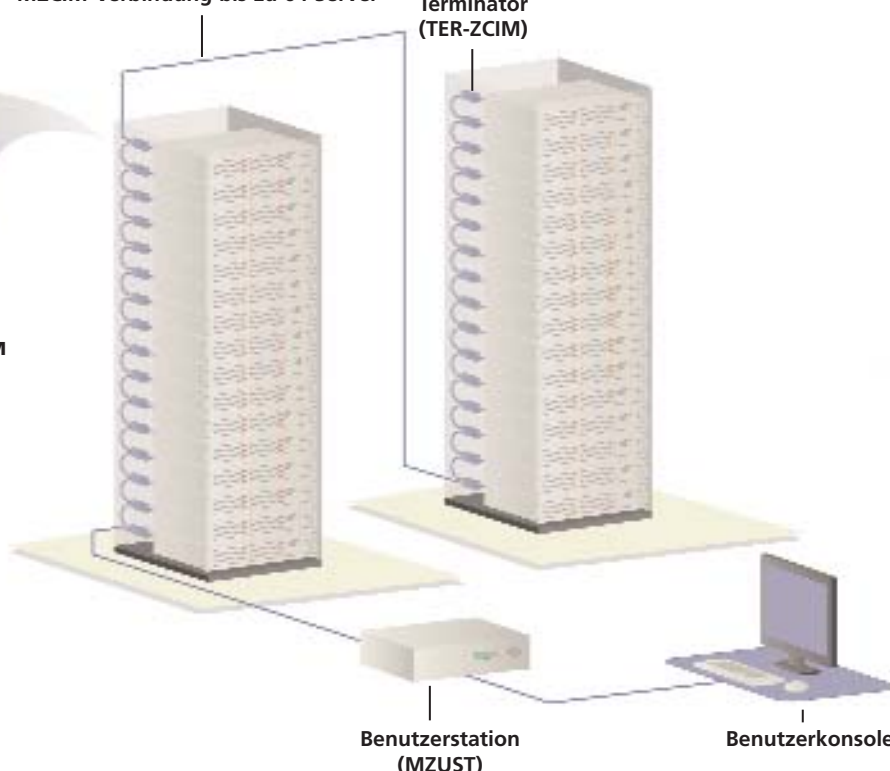
MZCIM-Verbindung bis zu 64 Server
